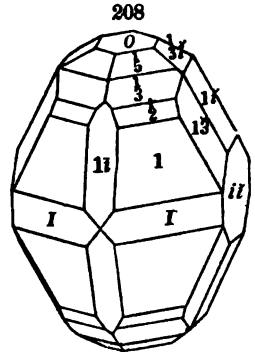
Sulphur.
